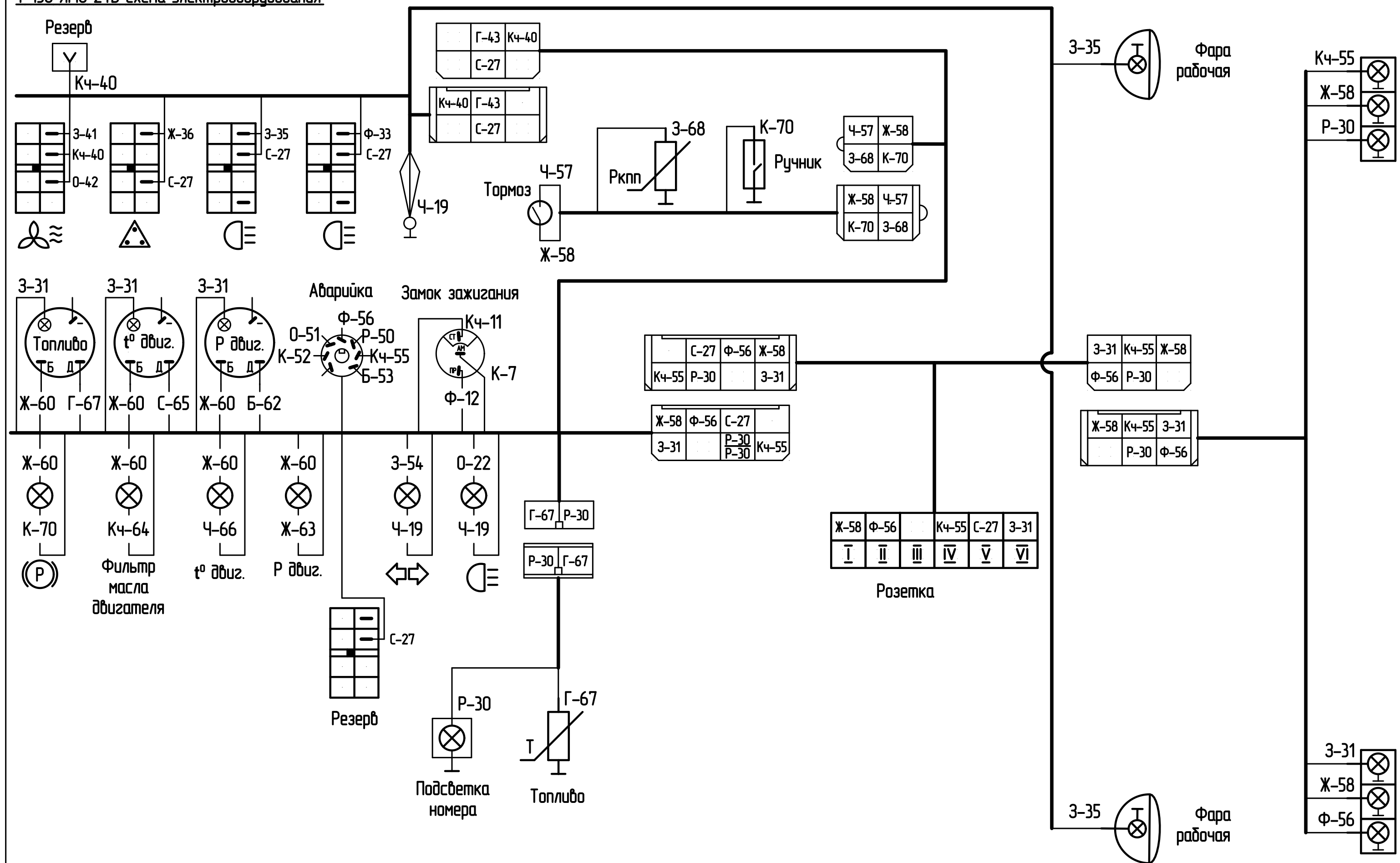
Т 150 ЯМЗ 24В схема электрооборудования
